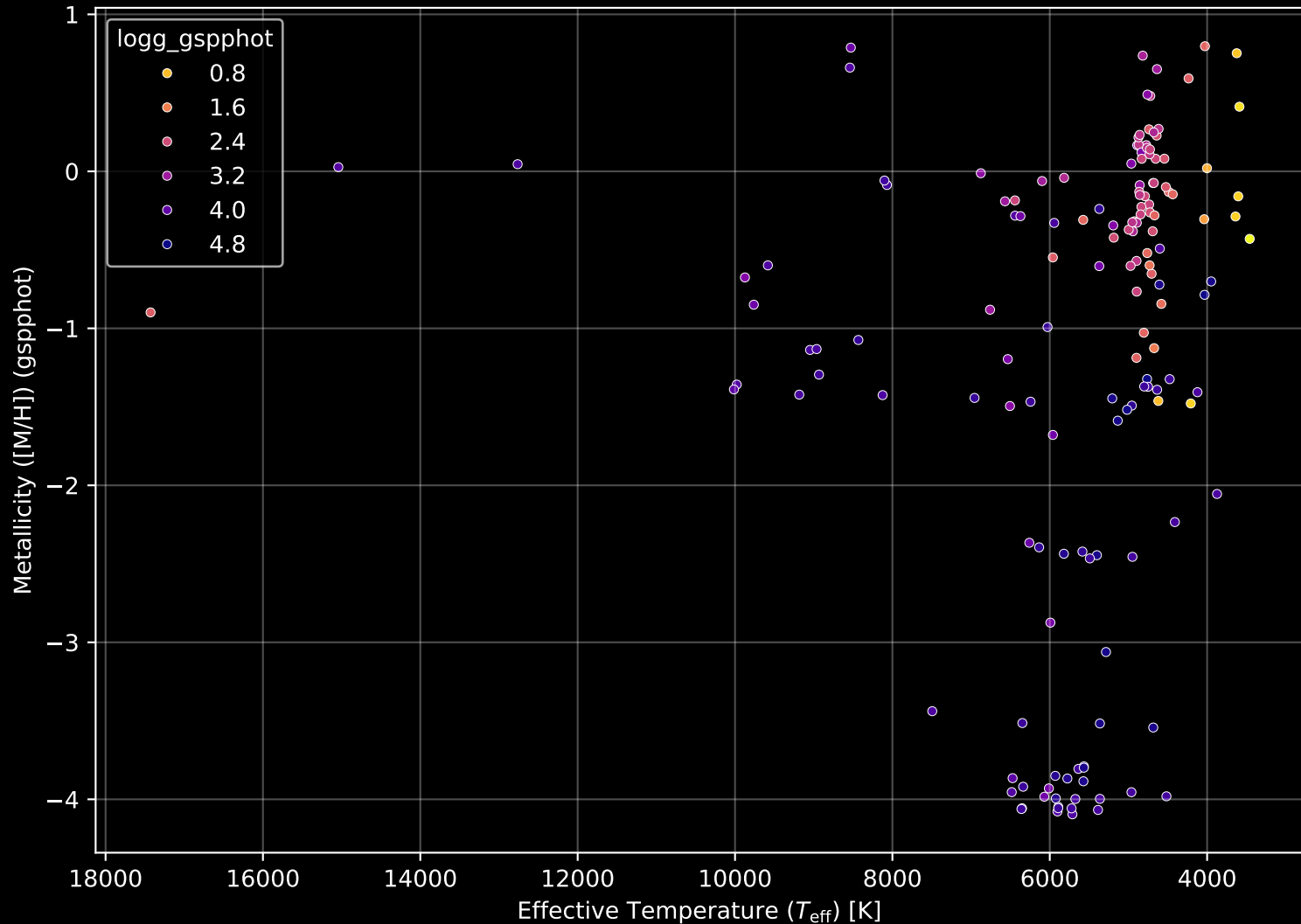
APOGEE DR17 Field: [006+04-O] Stellar Population Parameters (n= 154)
